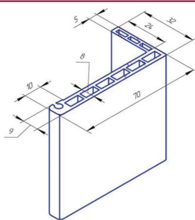
Добор телескопический L135
