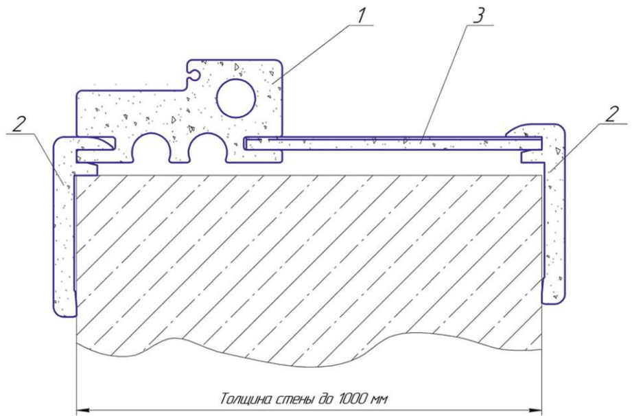
1 - Дверная коробка 80 2 - F наличник 3 - Добор прямой 5 мм
