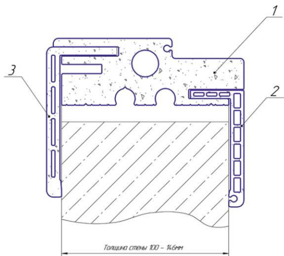
1 - Дверная коробка 80 2 - F наличник
