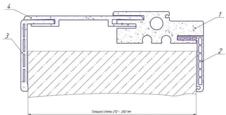
1 - Дверная коробка 100 2 - Наличник L32 3 - Наличник L42 4 - Добор E150
